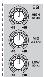
Fig. 2.5: La regulación de sonido de los canales estéreo de entrada
