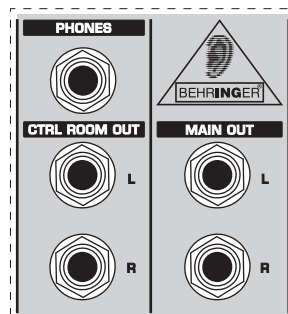
Fig. 2.9: Conexiones de mezcla de monitorización /mezcla principal
