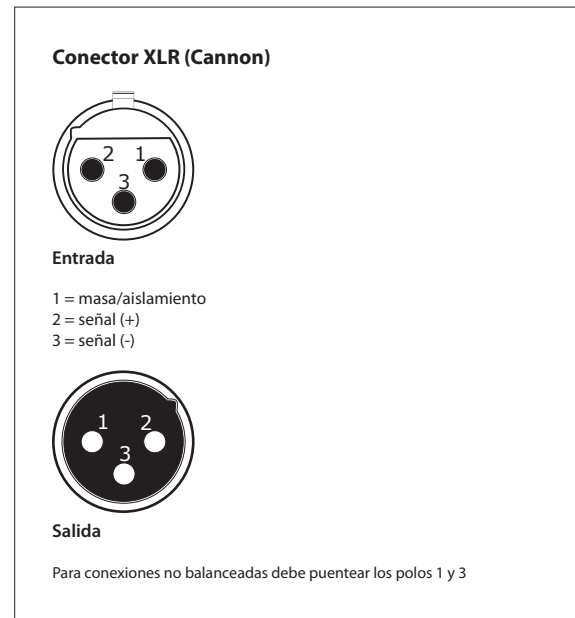
Fig. 3.1: Conexiones XLR
