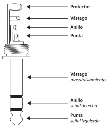
Fig. 3.4: Jack macho estéreo para auriculares
