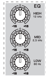
Fig. 2.2: La regulación de sonido de los canales mono de entrada
