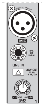
Fig. 2.1: Conexiones y reguladores de las entradas mic/line
