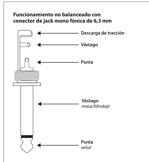
Fig. 3.2: Jack macho mono de 6,3 mm
